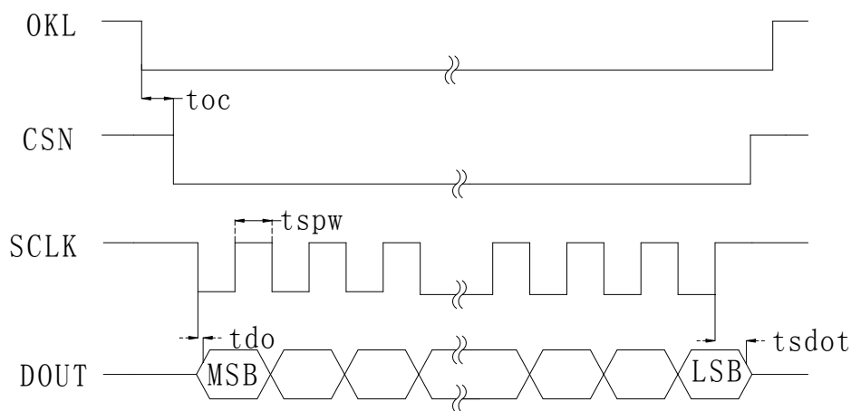
图 4 读时序
