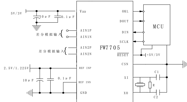
图 5 FW7705 的电路图
