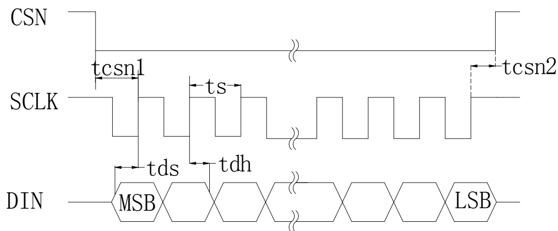
图 3 写时序
