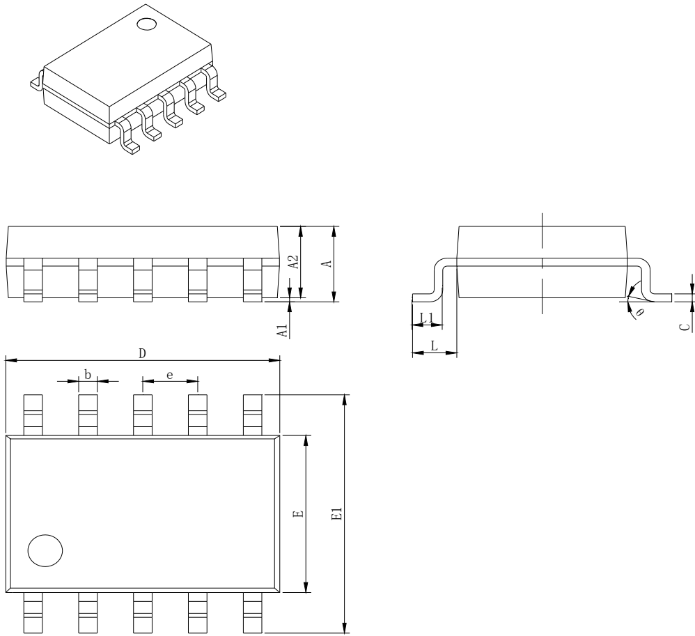
封装示意图 (SSOP10)
